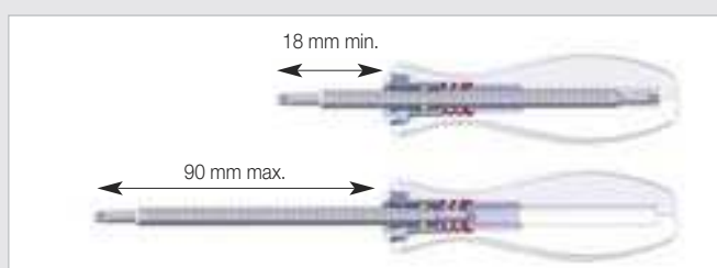
Mit dem SoftFinish®-telescopic Griff ist die Klingenslänge im Bereich von 18 – 90 mm variabel einstellbar.
